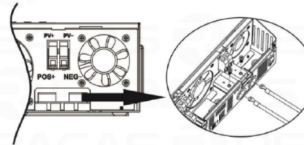
CONEXIÓN BATERÍAS-INVERSOR
