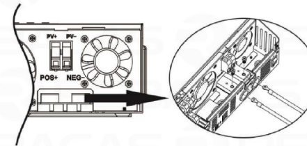
CONEXIÓN BATERÍAS-INVERSOR
