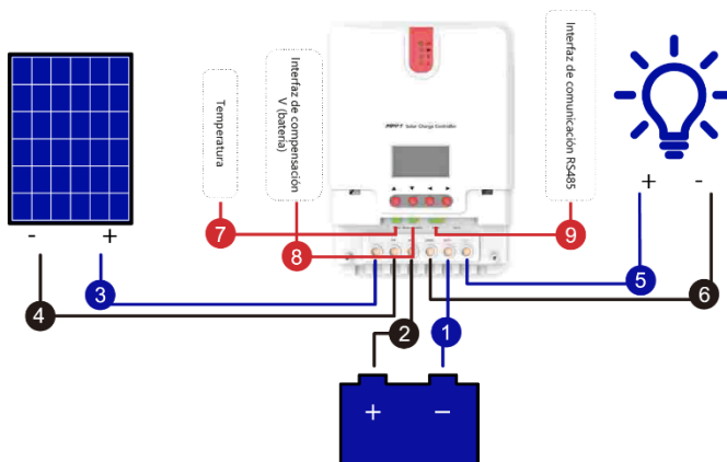
Fig 7. Cableado
