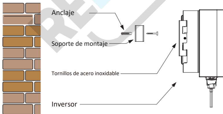
Imagen 4.4 Instalación del inversor
