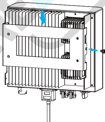
Imagen 4.6 Instalación del inversor
