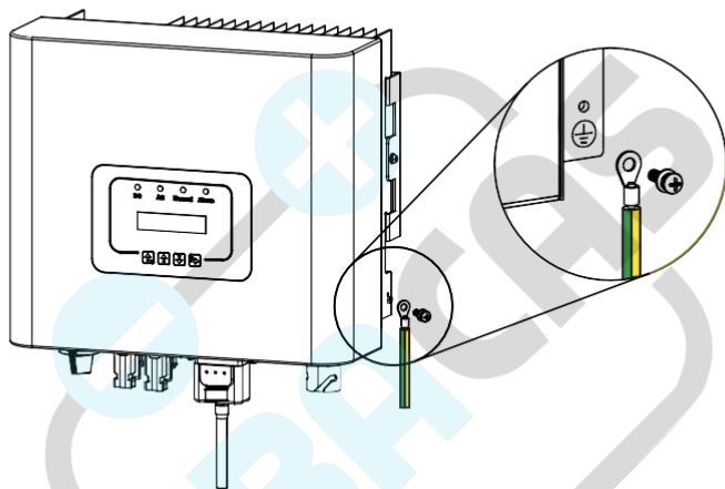
Imagen 5.11 La instalación del cable de tierra de la carcasa
