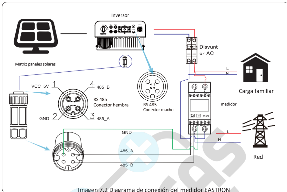
Imagen 7.2 Diagrama de conexión del medidor EASTRON
