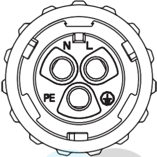
Imagen 5.9 Patrón de orificios del conector de AC
