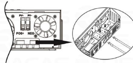
CONEXIÓN BATERÍAS-INVERSOR
